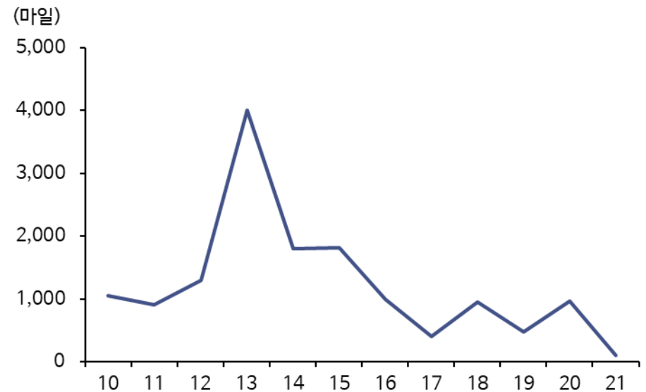
미국 송전망(345kV 이상) 설치 추이
